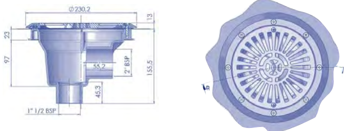
Донный слив с плоской решеткой
