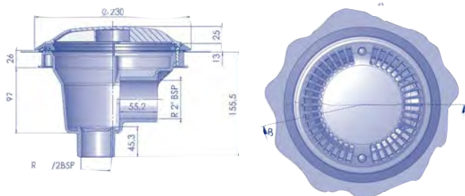
Донный слив с антивихревой решеткой
